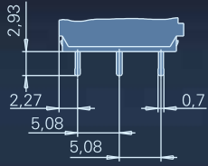
PCB terminal 0,7x0,5 mm, straight
