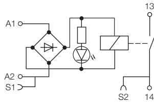
RB(R)111-24VUC
