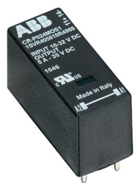
CR-P optocoupler
